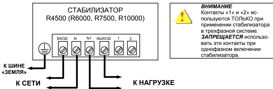
Рисунок 6.1 Схема подключения стабилизатора
