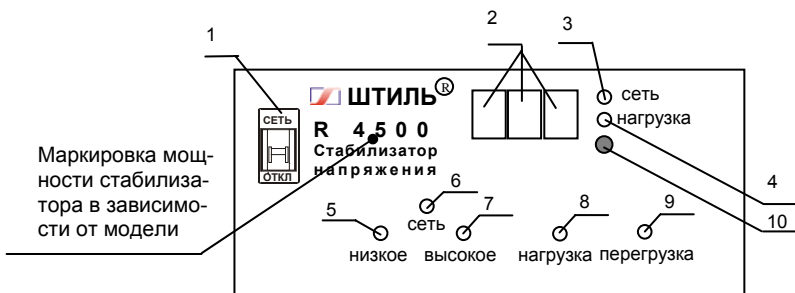
Рисунок 4.1 Передняя панель стабилизатора
