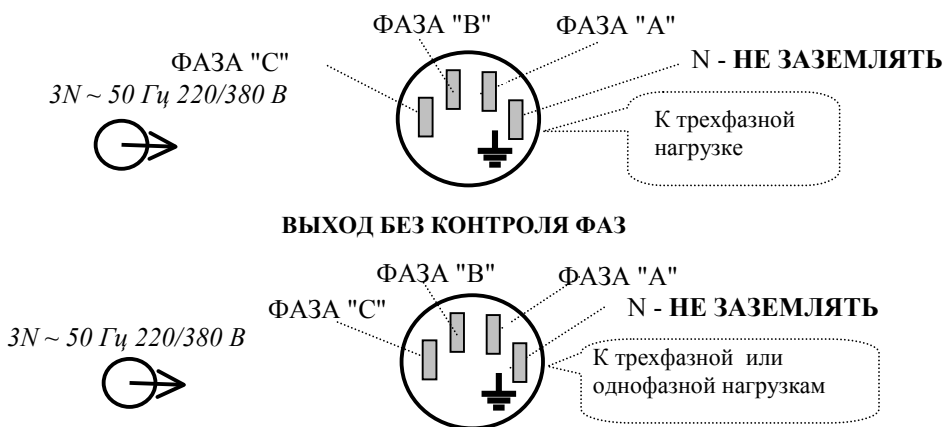
Рисунок 2 Схемы подключения нагрузки к стабилизатору R6000-3P (Вид на розетки со стороны задней панели стабилизатора)
