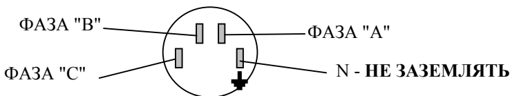
Рисунок 1 Схема подключения цепей питания стабилизатора R 6000-3 (Вид на розетку с внешней стороны)
