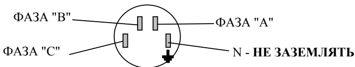
Рисунок 1 Схема подключения цепей питания стабилизатора R3600-3 (Вид на розетку с внешней стороны)
