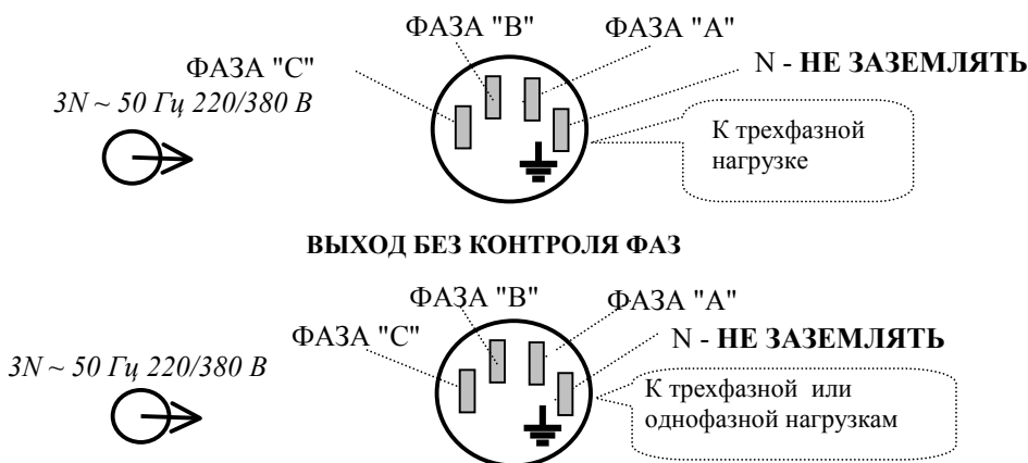
Рисунок 2 Схемы подключения нагрузки к стабилизатору R3600-3P (Вид на розетку со стороны задней панели стабилизатора)
