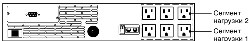
Рисунок 24. Сегменты нагрузки ИБП (для модели 120В)
