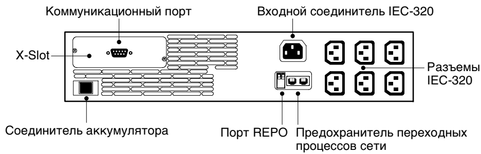
Рисунок 14. 700–2000 ВА, 230В, задняя панель
