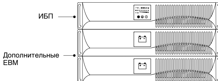
Рисунок 3. Монтаж ИБП с ЕВМ в стойку
