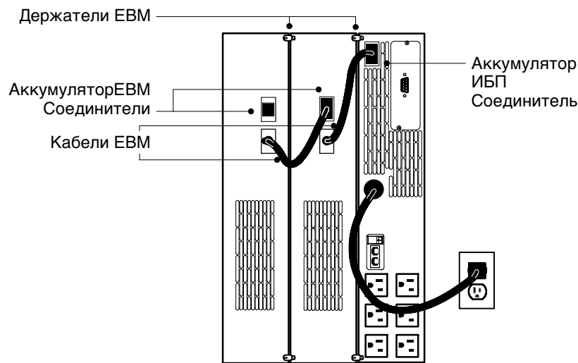
Рисунок 26. ЕВМ Соединители (для модели 120В)
