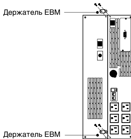
Рисунок 7. Установка держателей ЕВМ
