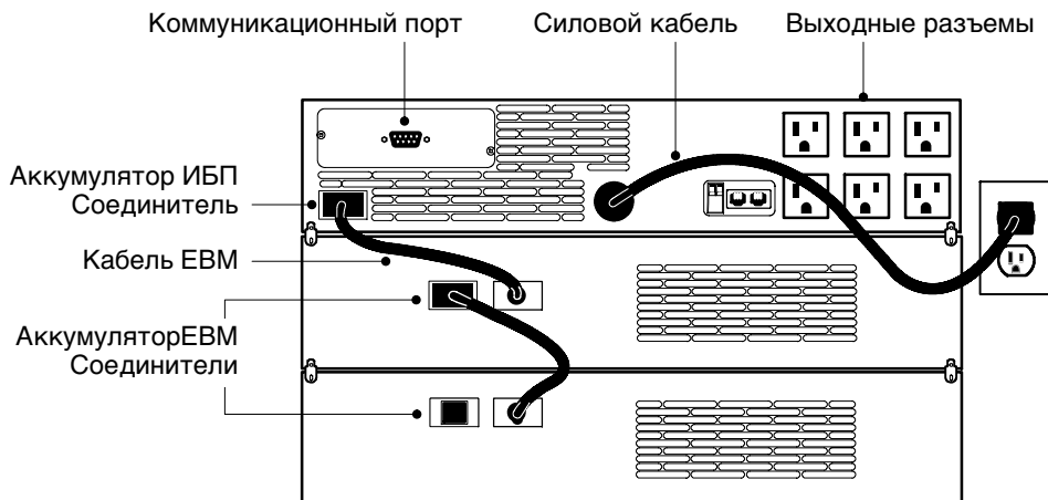
Рисунок 8. Типичная установка ИБП (для модели 120В)
