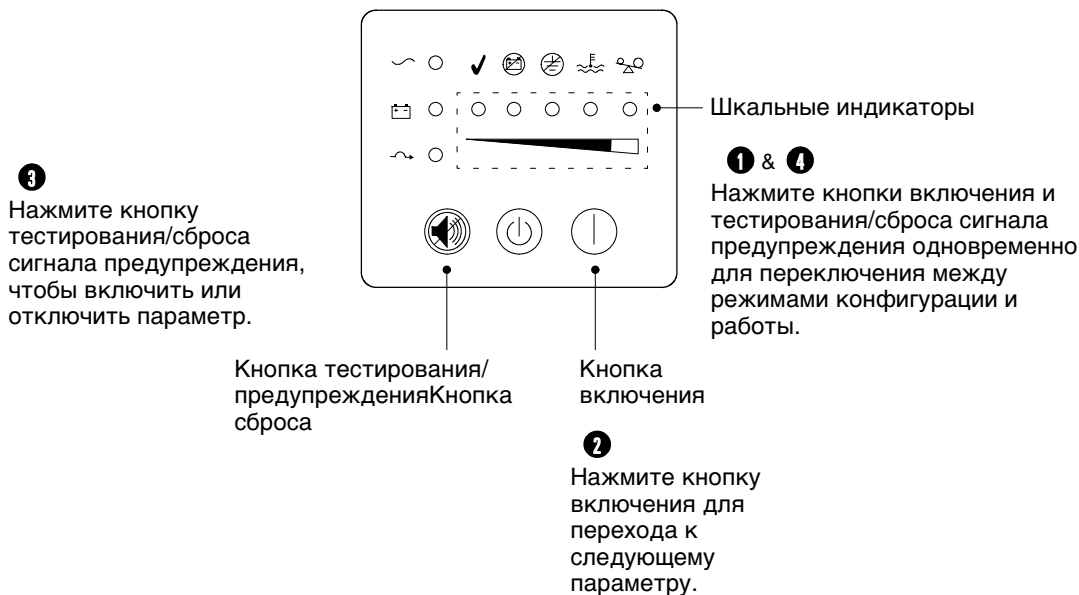
Рисунок 18. Использование режима конфигурации
