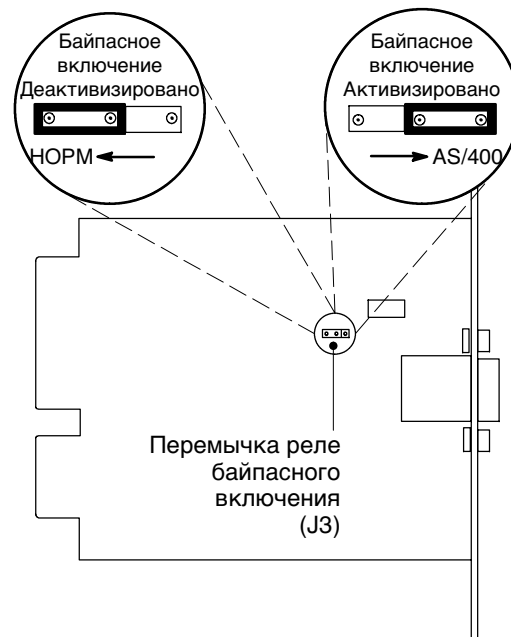
Рисунок 22. Переключатель реле байпасного включения
