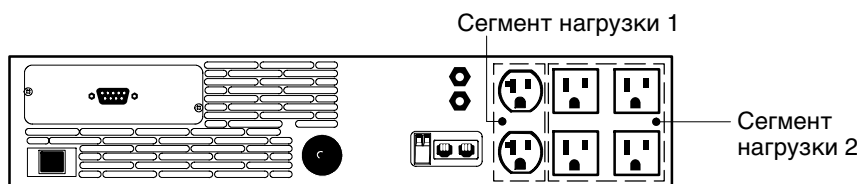
Рисунок 25. Сегменты нагрузки ИБП для: PW9125 2000 20R
